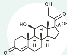
Cortisol C 21 H 30 O 5
